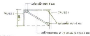
แบบขยาย 1 SCALE 1:25
