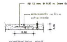
แบบขยายโครงสร้าง
