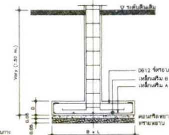
DETAIL FOR FOOTING F1 F2A
