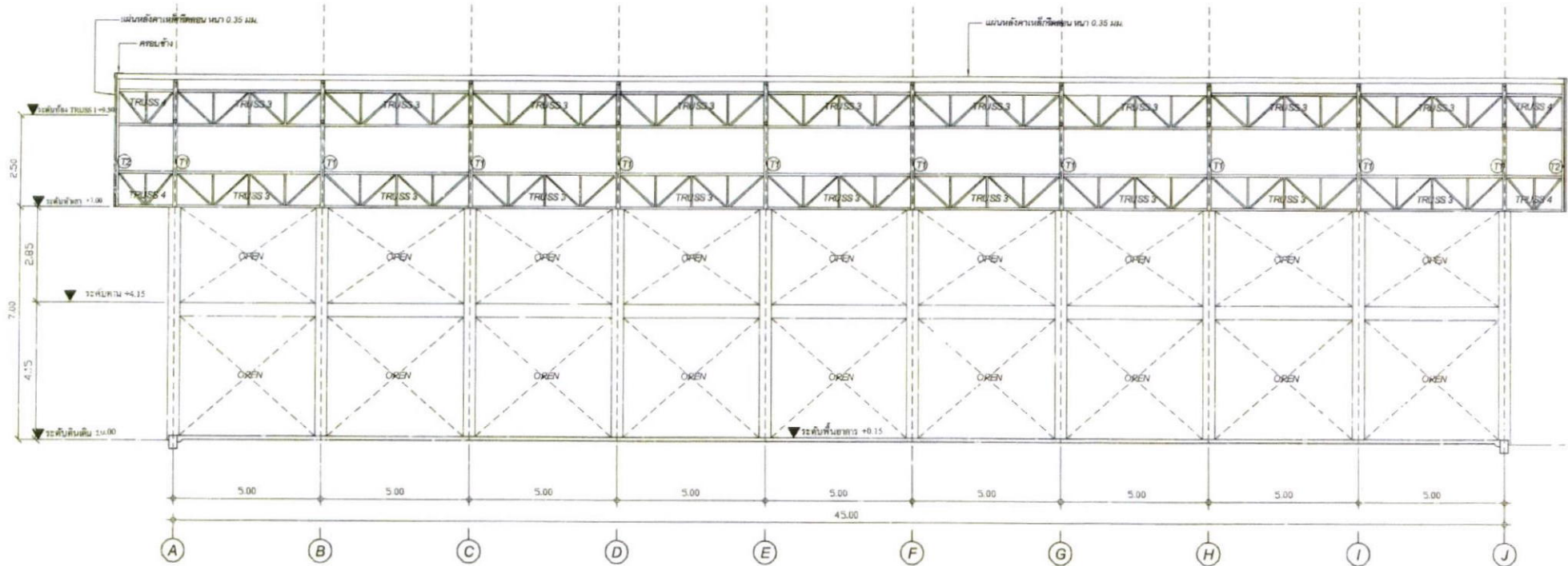
รูปตัด B-B SCALE 1:100
